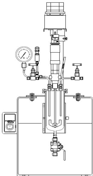
※800ml/1000ml/1500ml(φ96)仕様
